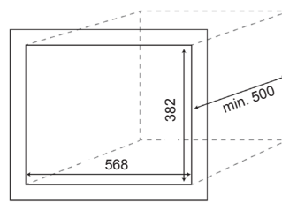
LKMW-2308 PRODUCT DIMENSION:(mm) 595 (w) x 388 (h) x 343.5 (d)
